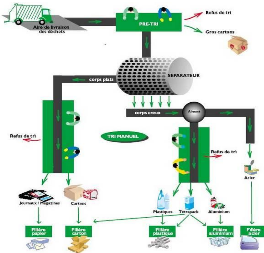
Schéma de fonctionnement d'un centre de tri
